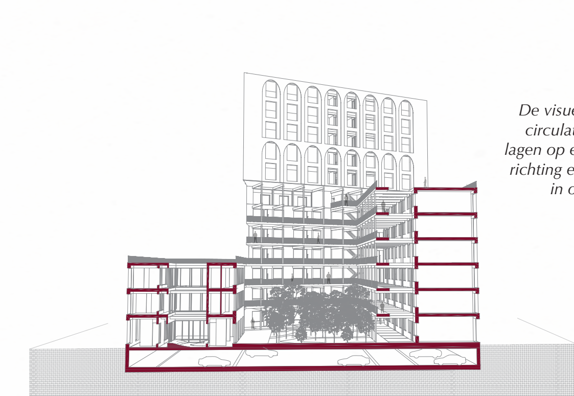
SNEDE AA'
