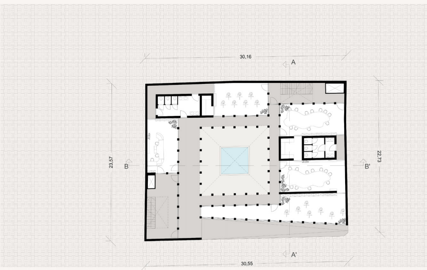
PLAN VERDIEP -1
